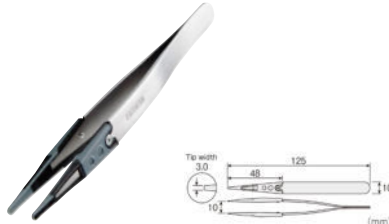
P-643-J ESD ELASTOMER TIP TWEEZERS
