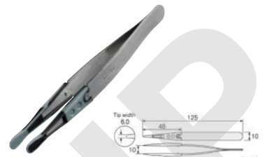
P-645-J ESD ELASTOMER TIP TWEEZERS
